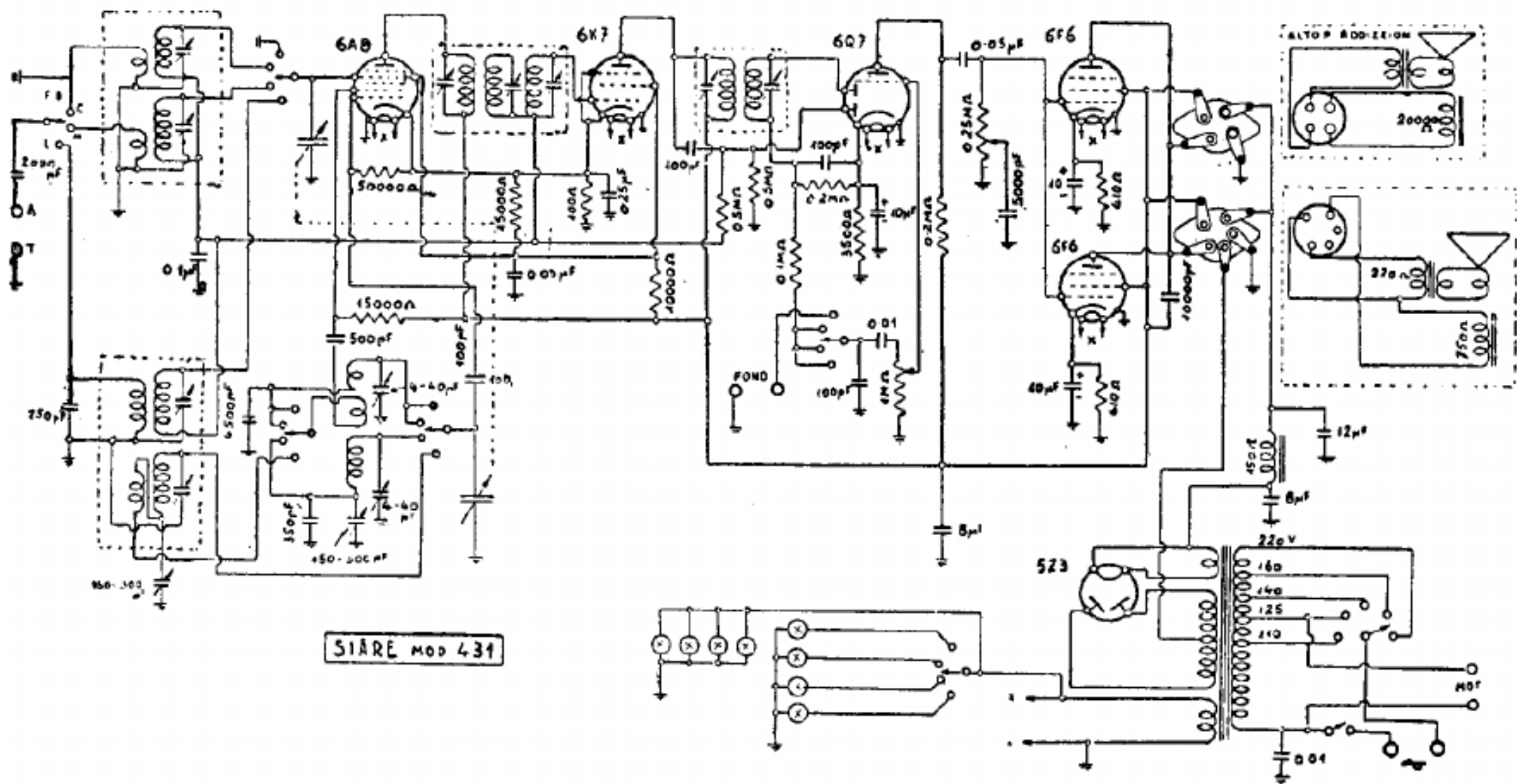
RADIO SIARE — Mod. « 431 C ». - Produzione 1937. Media frequenza: 468 k Hz.
